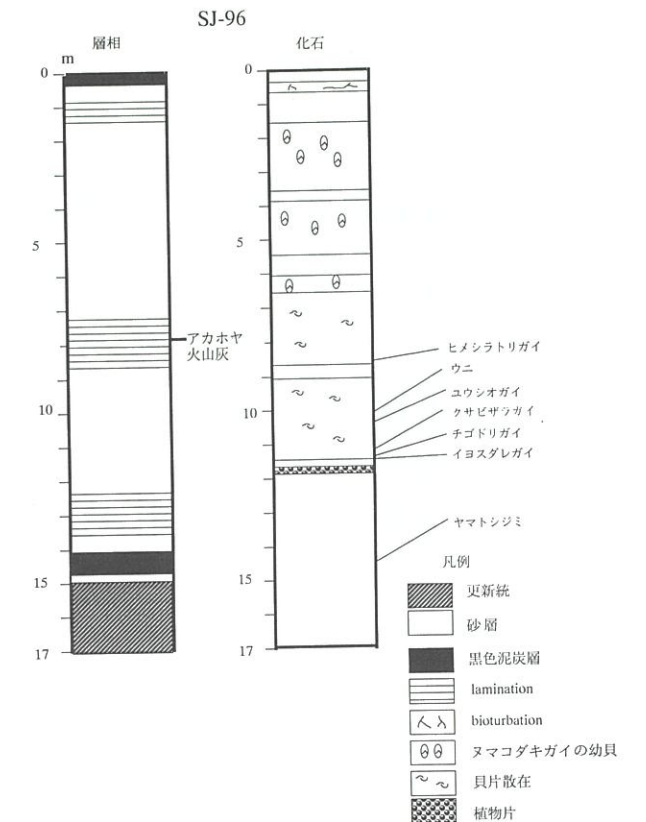
図4. 宍道湖ボーリングコア柱状図（SJ-96） Fig.4 Columnar section of the lithofacies sequence of Lake Shinji
