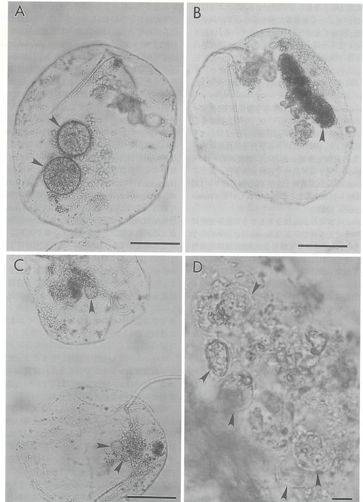
図11. ヤコウチュウ Noctiluca scintillans の食胞内容物。St.-4, 4月。A. カイアシ類の卵 (矢印), B. カイアシ類 (?) の糞粒 (矢印), C. Prorocentrum minimum (矢印), D. 食胞内にぎっしり詰まった P. minimum (矢印)。スケール: 100μm (A-C); 10μm (D)。 Fig.11. Contents in food vacuoles of Noctiluca scintillans . St.-4, April. A. Copepod eggs (arrowed), B. Fecal pellet of copepod (?) (arrowed), C. Prorocentrum minimum (arrowed), D. P. minimum packed in food vacuole (arrowed). Scale: 100μm (A-C); 10μm (D).
