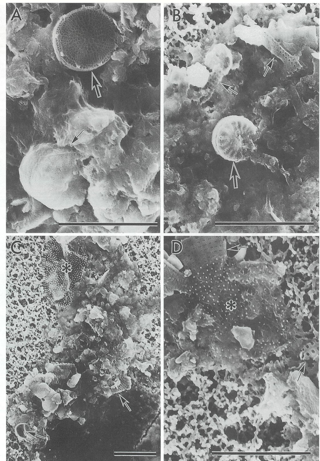
図9. Oithona davisae (成体雌) の消化管内容物。A-C. St.-4, 4月; D. St.-24, 4月。A. Cyclotella sp. (小さい矢印), Thalassiosira pseudonana (大きい矢印), B. Cyclotella sp. (大きい矢印), 珪藻類破片 (小さい矢印), C. Prorocentrum minimum (*), D. P. minimum (*), 珪藻類破片 (矢印)。スケール: 10µm。
