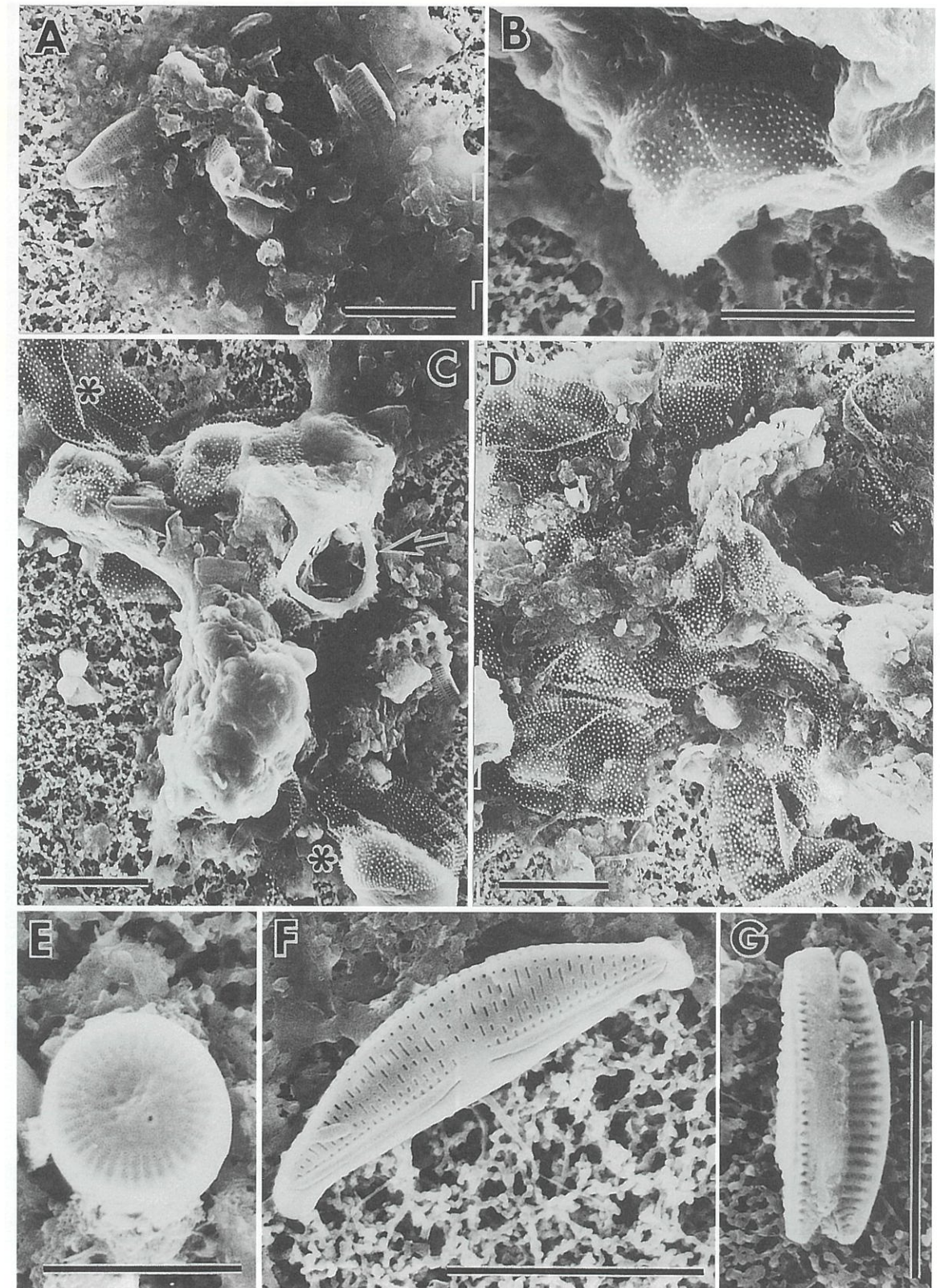
図3. Acartia hudsonica (成体雌) の消化管内容物. A-B. St.-4, 1月; C-G. St.-4, 4月. A. Navicula sp., B. Prorocentrum minimum , C. P. minimum (*), Ebria sp. (矢印), D. P. minimum , E. Cyclotella sp., F. Amphora sp., G. Nitschia sp. スケール: 10 \mu m (A-D, F, G), 5 \mu m (E).
