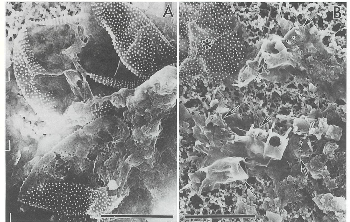
図7. Eurytemora pacifica (成体雄) の消化管内容物. St.-24, 4月. A. Prorocentrum minimum , B. P. minimum (*), Skeletonema costatum (矢印). スケール: 10 \mu m.
