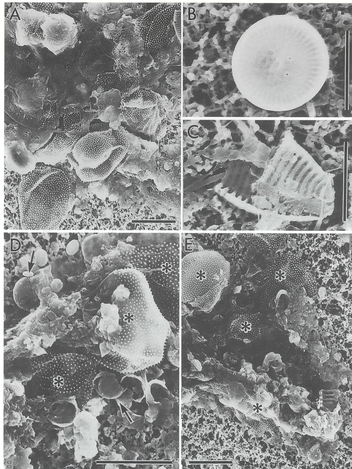
図8. Sinocalanus tenellus (成体雌) の消化管内容物。A-C. St.-4, 4月; D, E. St.-24, 4月。A. Prorocentrum minimum , B. Cyclotella choctawhatcheeana , C. Nitzschia sp., D. P. minimum (*), Thalassiosira pseudonana (矢印), E. P. minimum (*), 珪藻類破片。スケール: 10µm (A, D, E); 5µm (B, C)。
