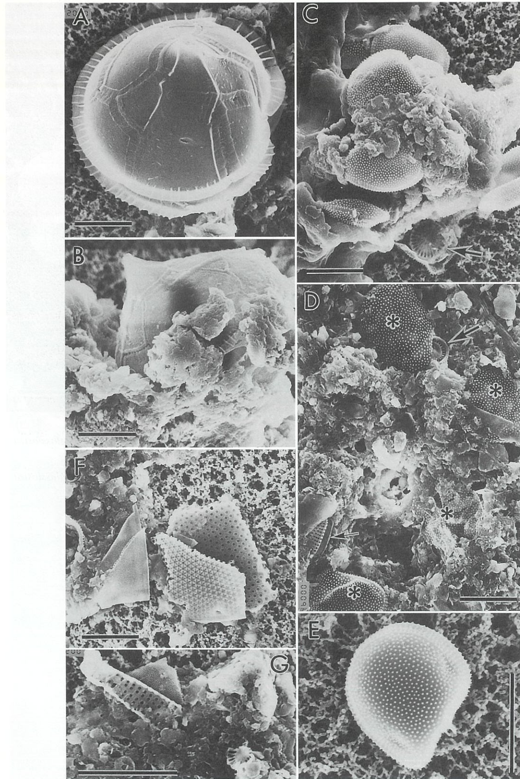
図6. Eurytemora pacifica (成体雌) の消化管内容物. St.-4, 1月. A, B. Protoperidinium sp.?, C. Prorocentrum minimum , Cyclotella sp. (矢印), D. P. minimum (*), Cyclotella sp. (大きい矢印), Neodelphineis pelagica (小さい矢印), E. P. minimum , F. 珪藻類の破片, G. Neodelphineis pelagica . スケール: 10 \mu m.
