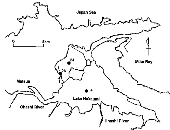
図1. 中海におけるプランクトンの採集定点。
