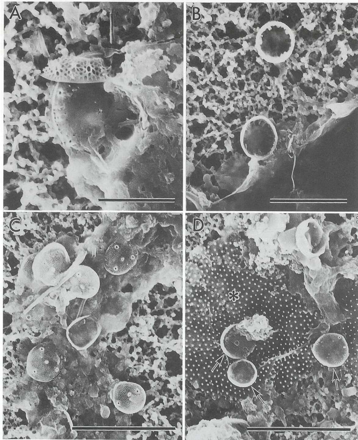
図10. Oithona davisae (成体雌) の消化管内容物。A, B. St.-4, 7月, C, D. St.-4, 9月。A. Skeletonema costatum , B. Cyclotella sp., C. Minidiscus comicus , D. Prorocentrum minimum (*), M. comicus (矢印)。スケール: 10μm。 Fig.10. Gut contents of Oithona davisae (adult female). A, B. St.-4, July; C, D. St.-4, September. A. Skeletonema costatum , B. Cyclotella sp., C. Minidiscus comicus , D. Prorocentrum minimum (*), M. comicus (arrowed). Scales: 10μm.
