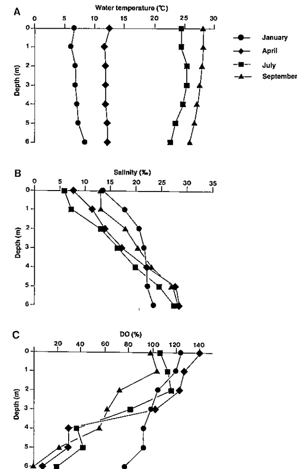
図2. 中海の定点4における水温 (A)、塩分 (B)、溶存酸素 (C) の鉛直分布。
