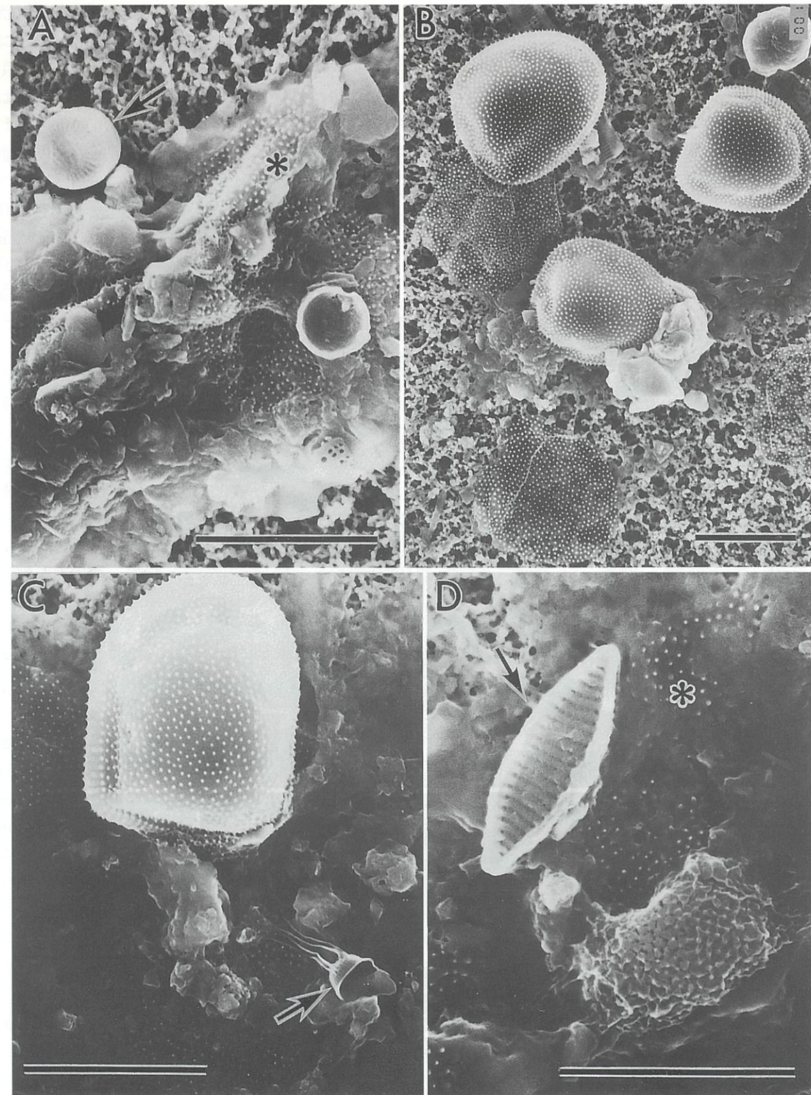
図4. Acartia hudsonica (成体雌) の消化管内容物. St.-24, 4月. A. Prorocentrum minimum (*), Cyclotella sp. (矢印), B. P. minimum , C. P. minimum , Skeletonema costatum (矢印), D. P. minimum (*), Nitschia sp. (矢印). スケール: 10 \mu m.
