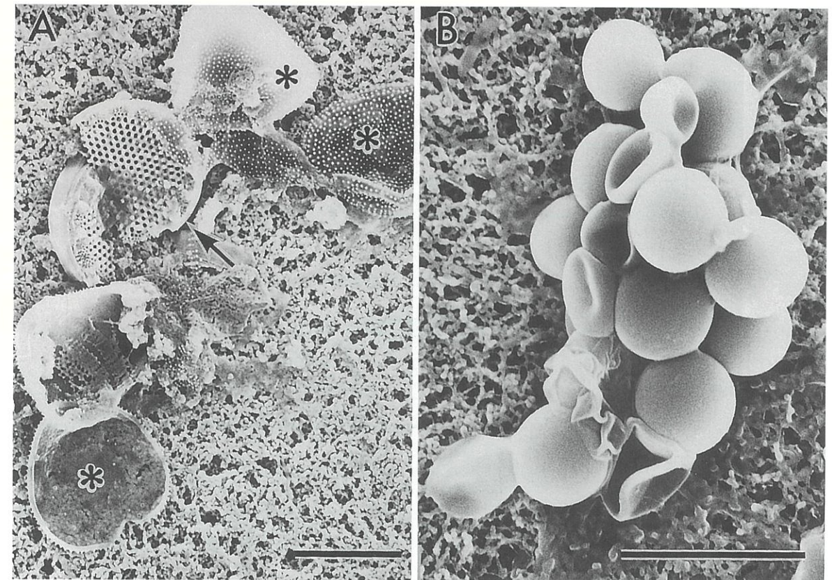
図5. Acartia sinjiensis (成体雌) の消化管内容物. St.-26, 9月. A. Prorocentrum minimum (*), Thalassiosira tenera (矢印), B. Bacteria? スケール: 10 \mu m.
