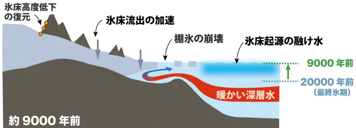
図 4：ドロンシングモードランドにおける東南極氷床融解メカニズムの模式図。
